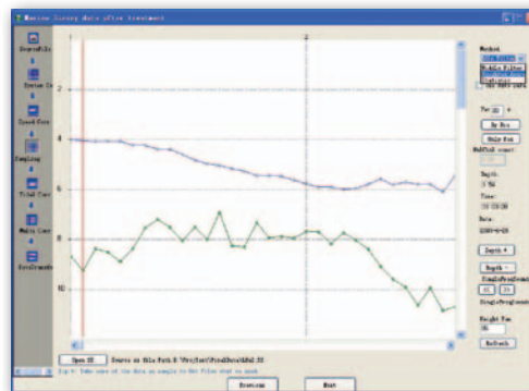
Pomiar echosondą dwuczęstotliwościową pozwala na monitorowanie dwóch obrazów dna zbiornika
